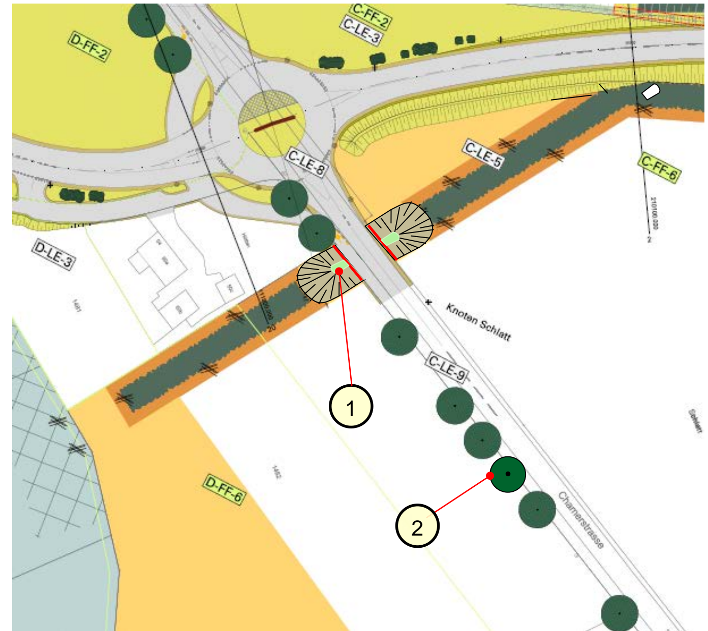
Abb. 1.2 Kleintierdurchlass
