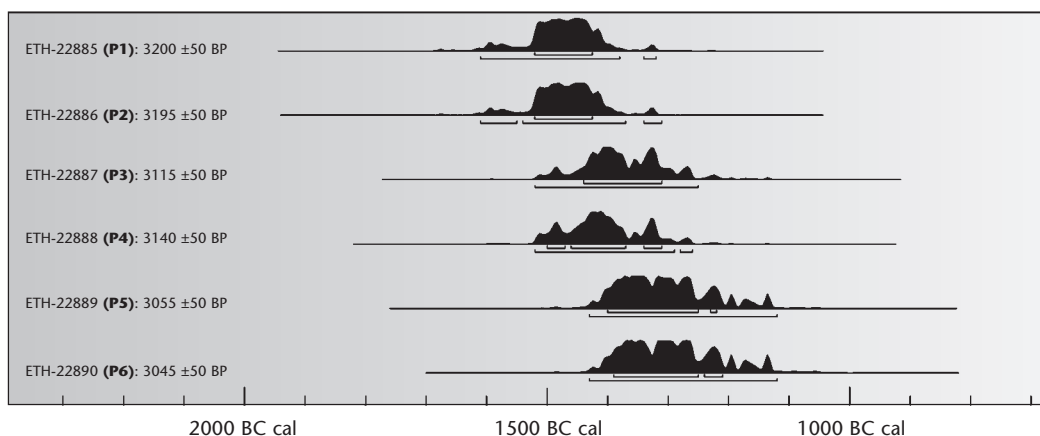
Abb. 100 Steinhausen-Chollerpark, US. Datierung der Abies-Mittelkurve 2520. a: Lage der sechs entnommenen Jahrringsequenzen (P1–P6) für die C14-Analyse. b: Tabellarische Zusammenstellung der Ergebnisse. c: Lage der C14-Rohdaten auf der Kalibrationskurve (Radiocarbon 40, 1998). d: Darstellung der Wahrscheinlichkeitsdichten für die verschiedenen kalibrierten C14-Datenspannen (Programm: OxCal 3.5).
