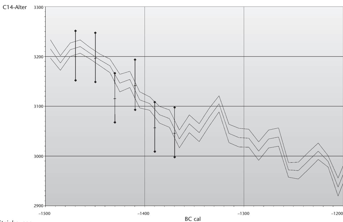
Abb. 100 Steinhausen-Chollerpark, US. Datierung der Abies-Mittelkurve 2520. a: Lage der sechs entnommenen Jahrringsequenzen (P1–P6) für die C14-Analyse. b: Tabellarische Zusammenstellung der Ergebnisse. c: Lage der C14-Rohdaten auf der Kalibrationskurve (Radiocarbon 40, 1998). d: Darstellung der Wahrscheinlichkeitsdichten für die verschiedenen kalibrierten C14-Datenspannen (Programm: OxCal 3.5).
