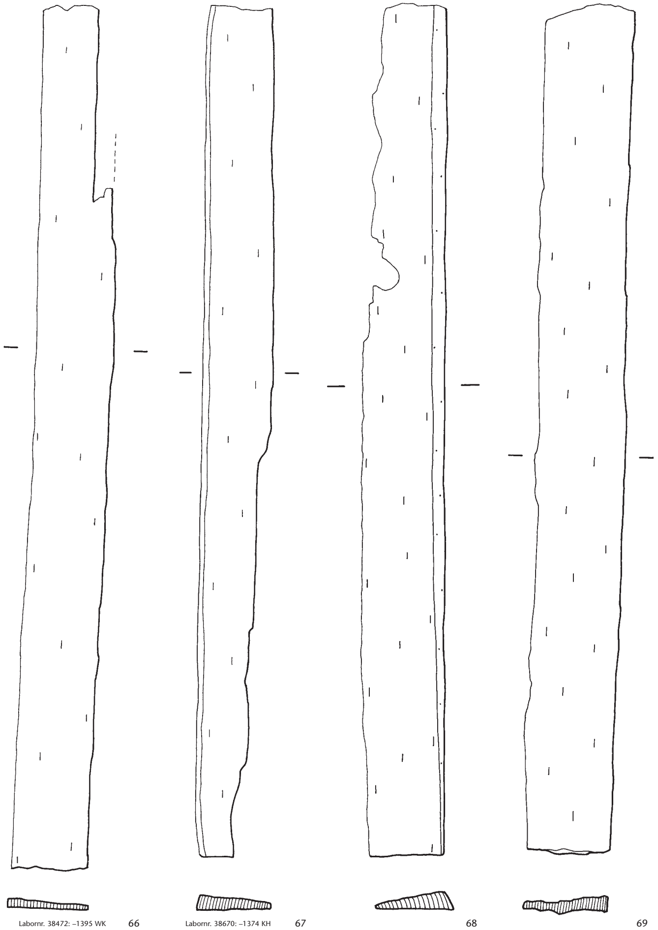
Tafel 14 Steinhausen ZG-Chollerpark, US. Bretter und Bohlen (66-69). Weisstanne (66-69). M. 1:10.
