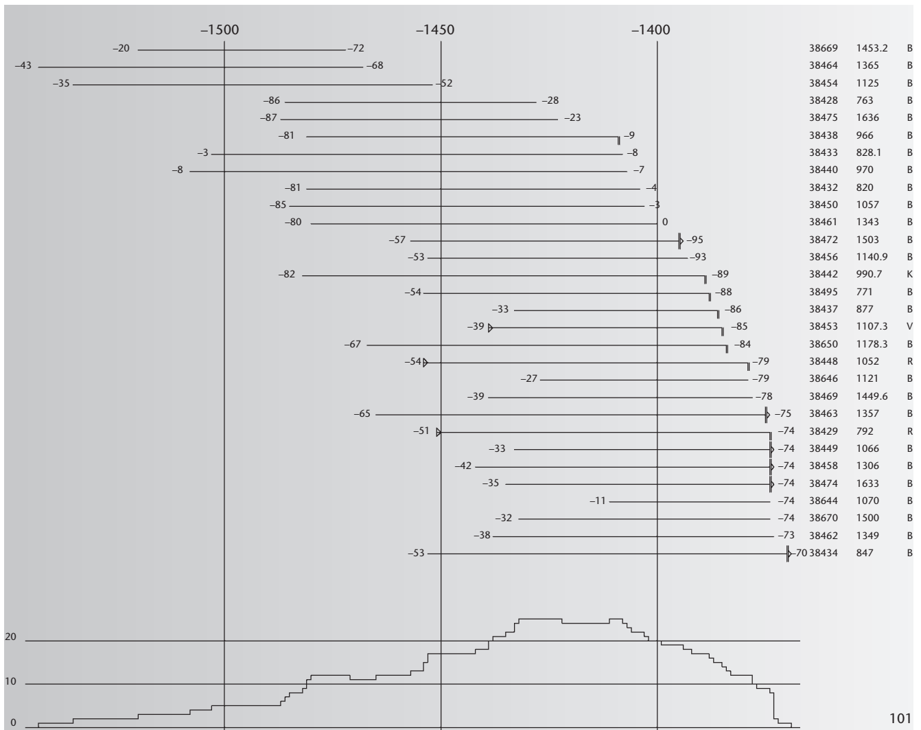
Abb. 101 Steinhausen-Chollerpark, US. Balkendiagramm mit den datierten und in die Abies-Mittelkurve 2520 integrierten Weisstannen. In der rechten Spalte finden sich Labornr., Holznr. und Querschnittform. Zu den Abkürzungen siehe Abb. 37. Unter dem Balkendiagramm ist die Belegungsdichte graphisch umgesetzt.
