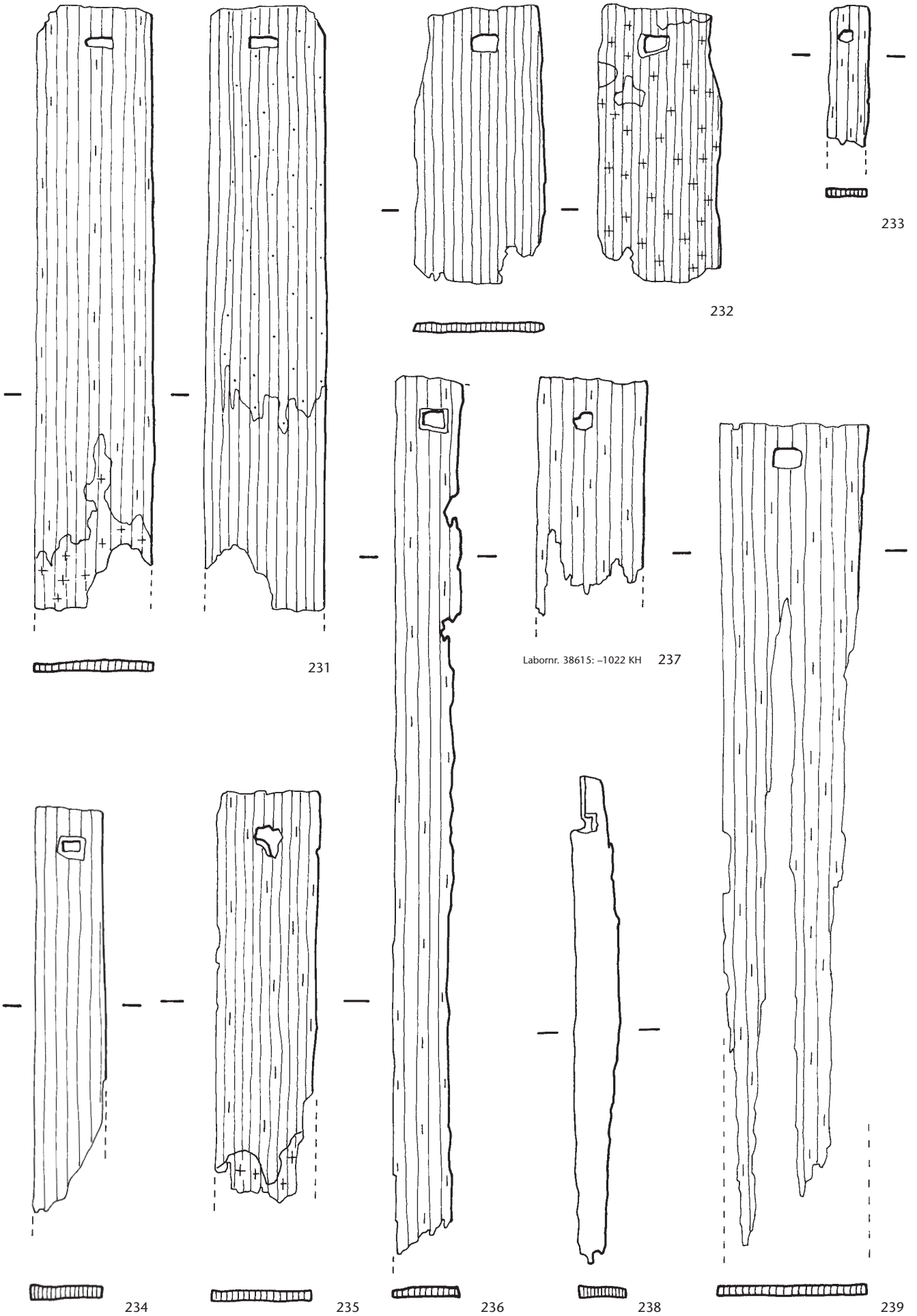
Tafel 36 Steinhausen ZG-Chollerpark, OS. Schindeln (231–239). Weissstanne (231–239). M. 1:10.
