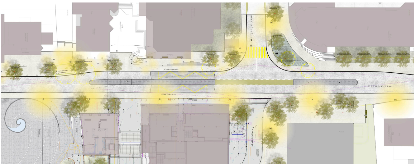
Abb. 14 Gestaltungskonzept Chamerstrasse, Stand 03.09.2021 (Quelle: Benedikt Stähli Landschaftsarchitekt BSLA)
