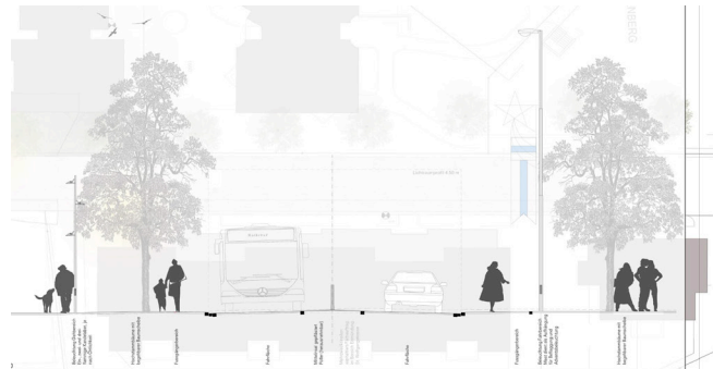
Abb. 16 Schnitt Gestaltungskonzept Chamerstrasse, Stand 03.09.2021 (Quelle: Benedikt Stähli Landschaftsarchitekt BSLA)
