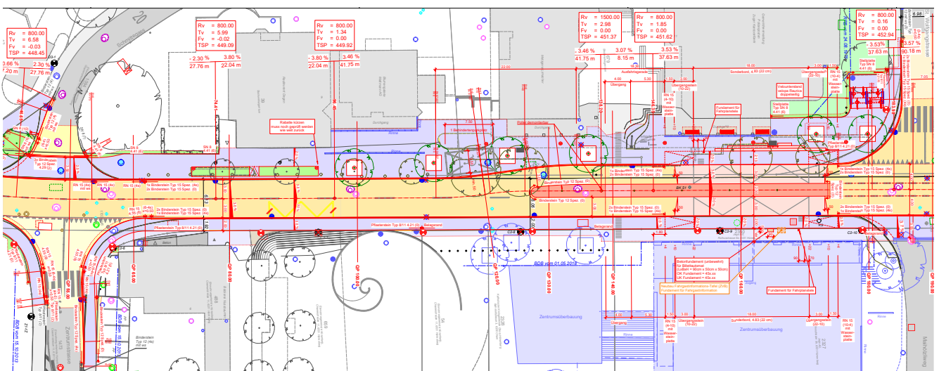
Abb. 15 Aufwertung Chamerstrasse Strassenbau Auflageprojekt, Stand 03.09.2021 (Quelle: TBA Kanton Zug)
