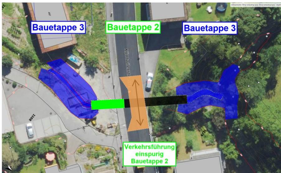
Verkehrsführung einspurig mit Lichtsignalanlage auf der Küntwilerstrasse (orange Fläche)
