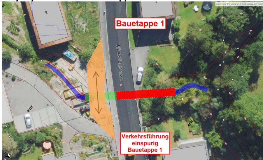
Verkehrsführung einspurig mit Lichtsignalanlage neben der Küntwilerstrasse (orange Fläche)
