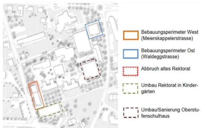
Situationsplan Schulareal Waldegg inkl. Neubauten
