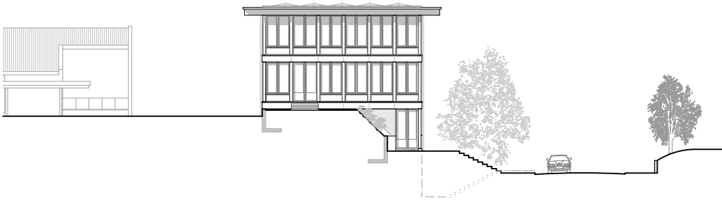
Nordfassade
