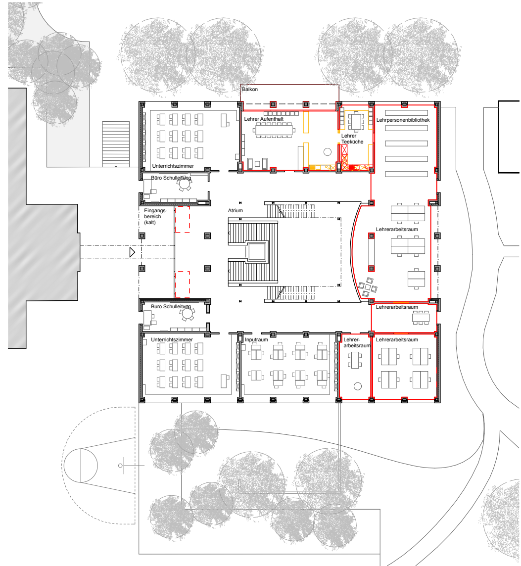
1. Obergeschoss
