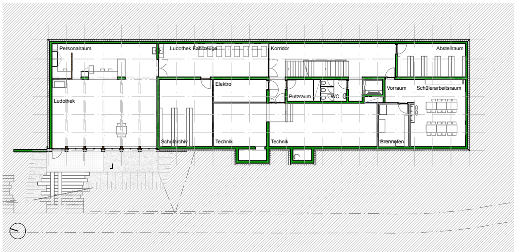
Untergeschoss
