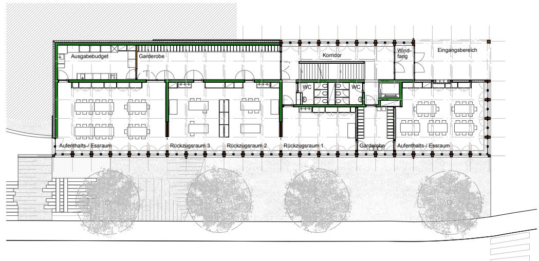
Erdgeschoss
