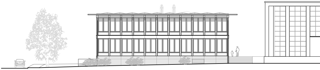
Nordfassade
