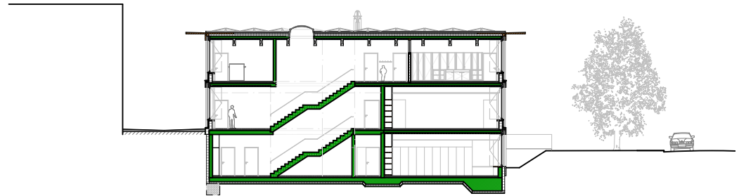
Querschnitt Treppenhaus
