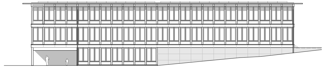
Ostfassade
