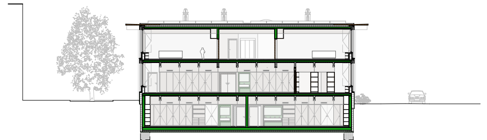
Querschnitt Unterrichtsräume
