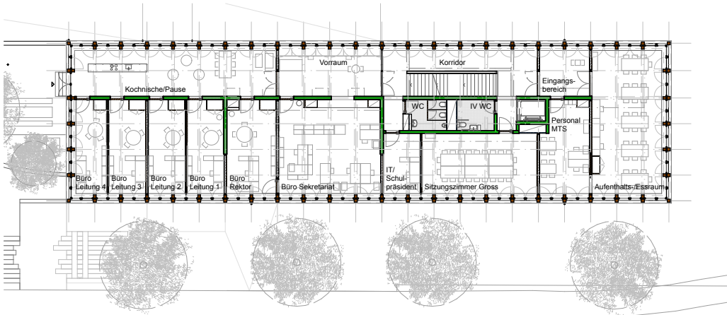
1. Obergeschoss
