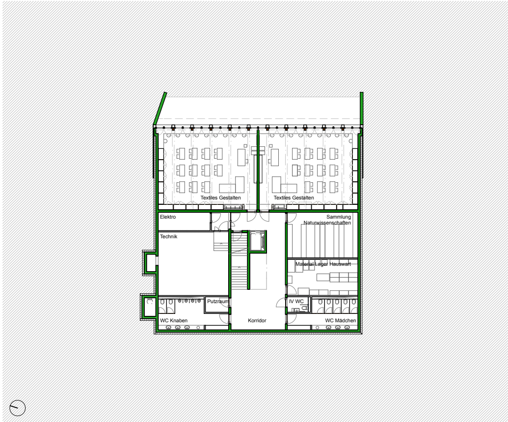
Untergeschoss
