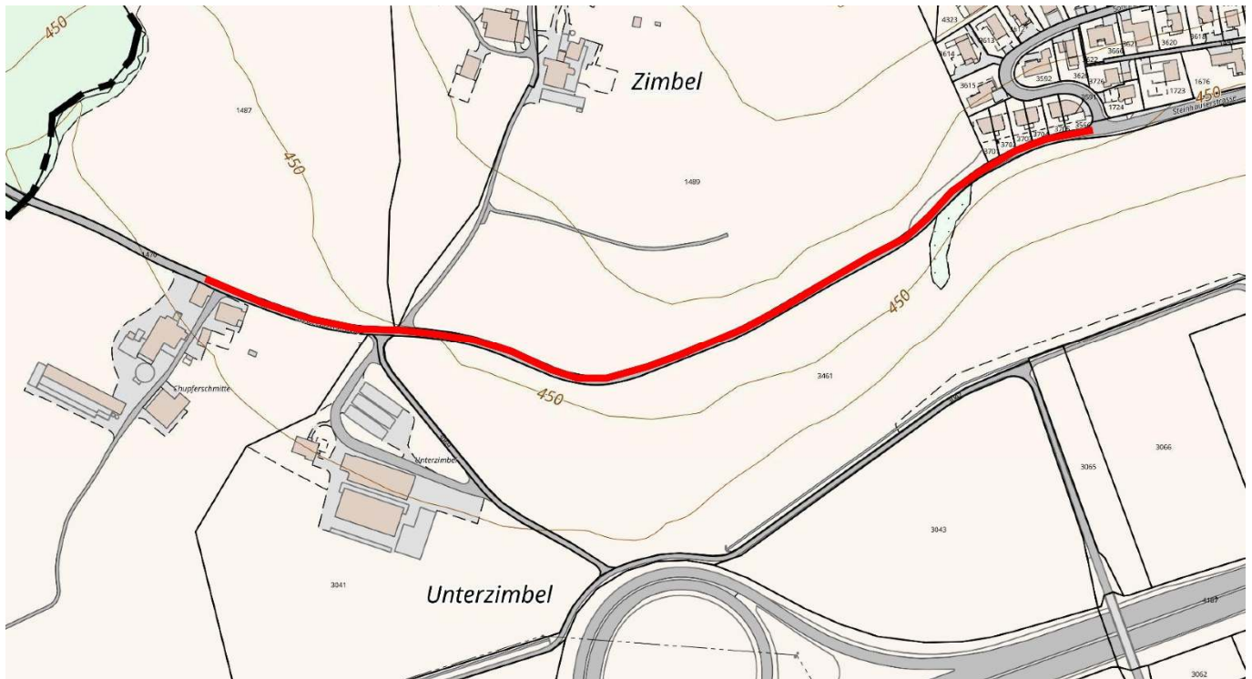
Sanierungsabschnitt Steinhauserstrasse
