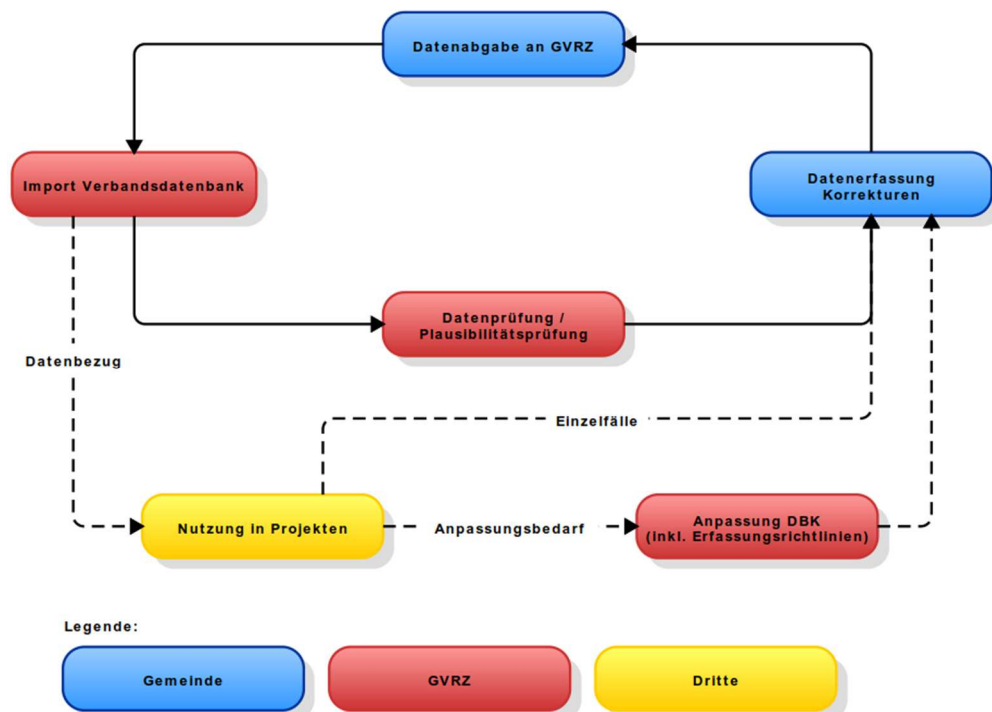
Abbildung 5: Verbesserungskreislauf
