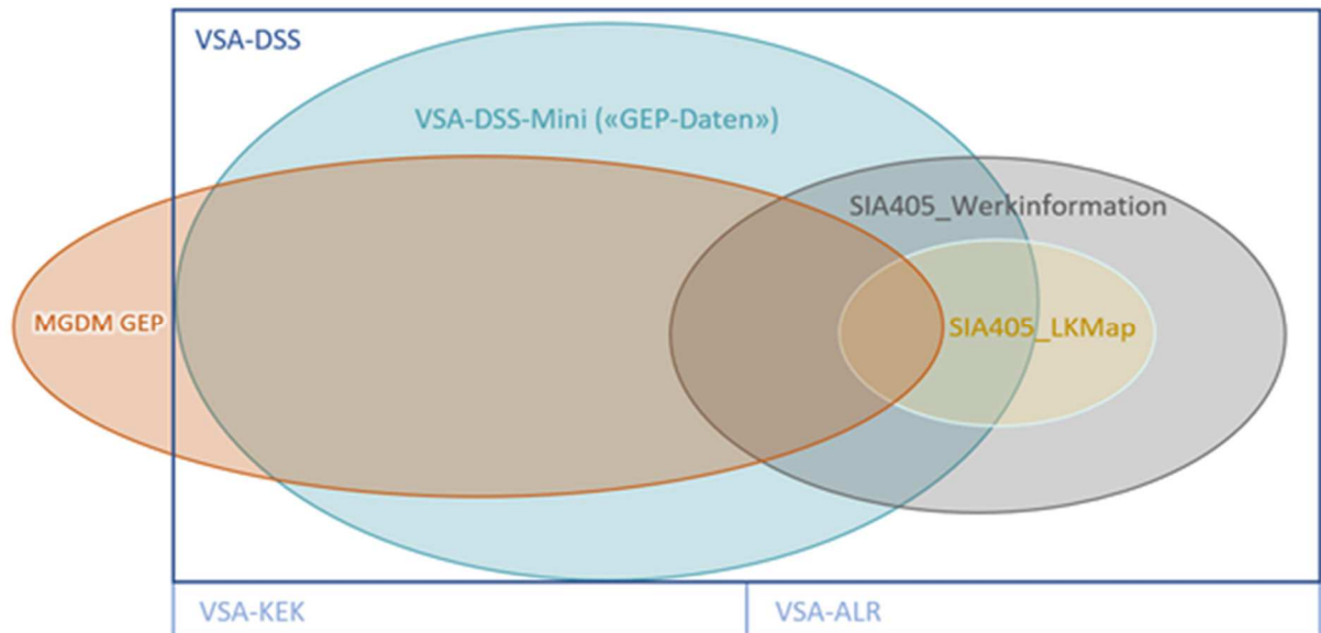
Abbildung 1: Inhaltlicher Umfang und Überschneidung eines Teils der beschriebenen Datenmodelle (seit der Version 2020 der Datenmodelle ist VSA-ALR nicht mehr als Erweiterung modelliert, sondern direkt in die VSA-DSS integriert)
