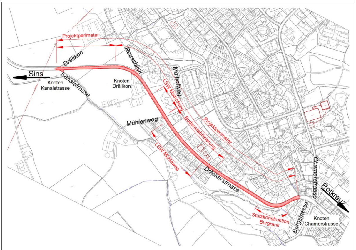
Übersichtsplan zur Sanierung der Drälikerstrasse in Hünenberg.
